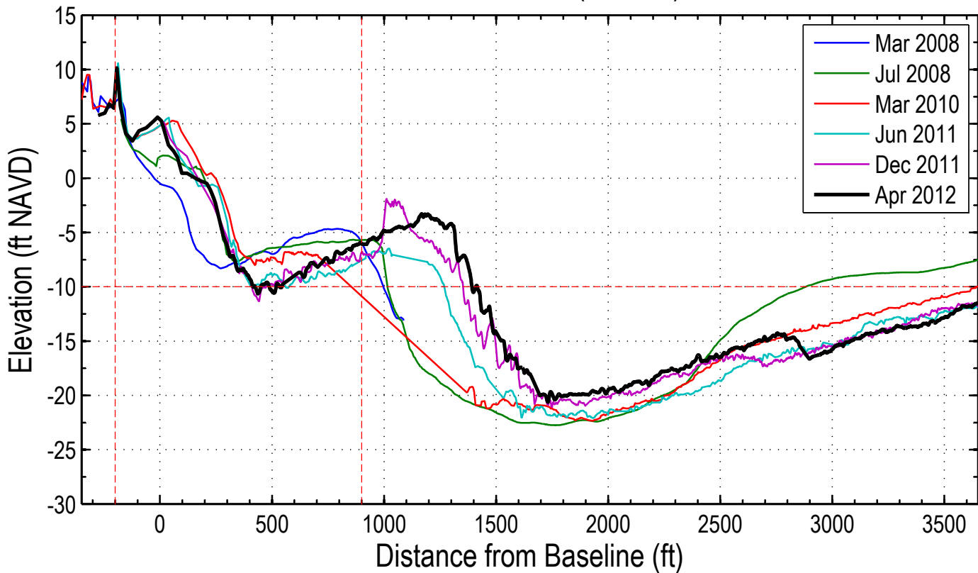
Station: 328+00 (106+00)
