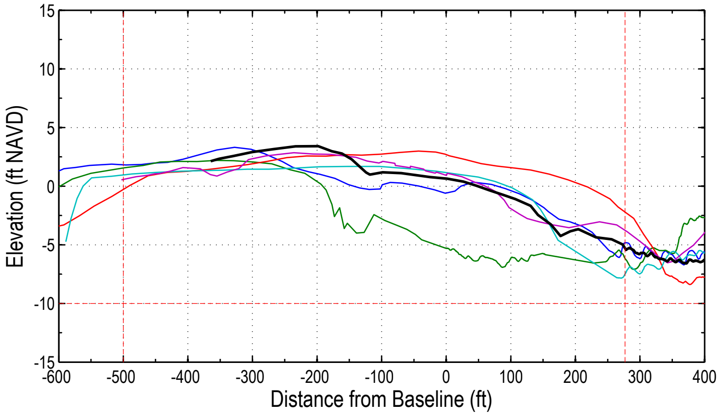
Station: 0+00
