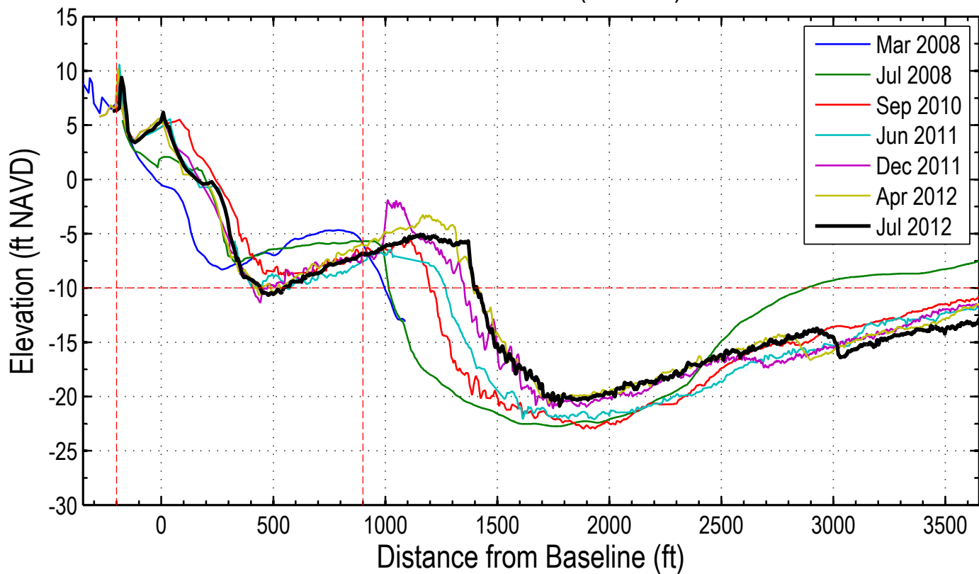
Station: 328+00 (106+00)
