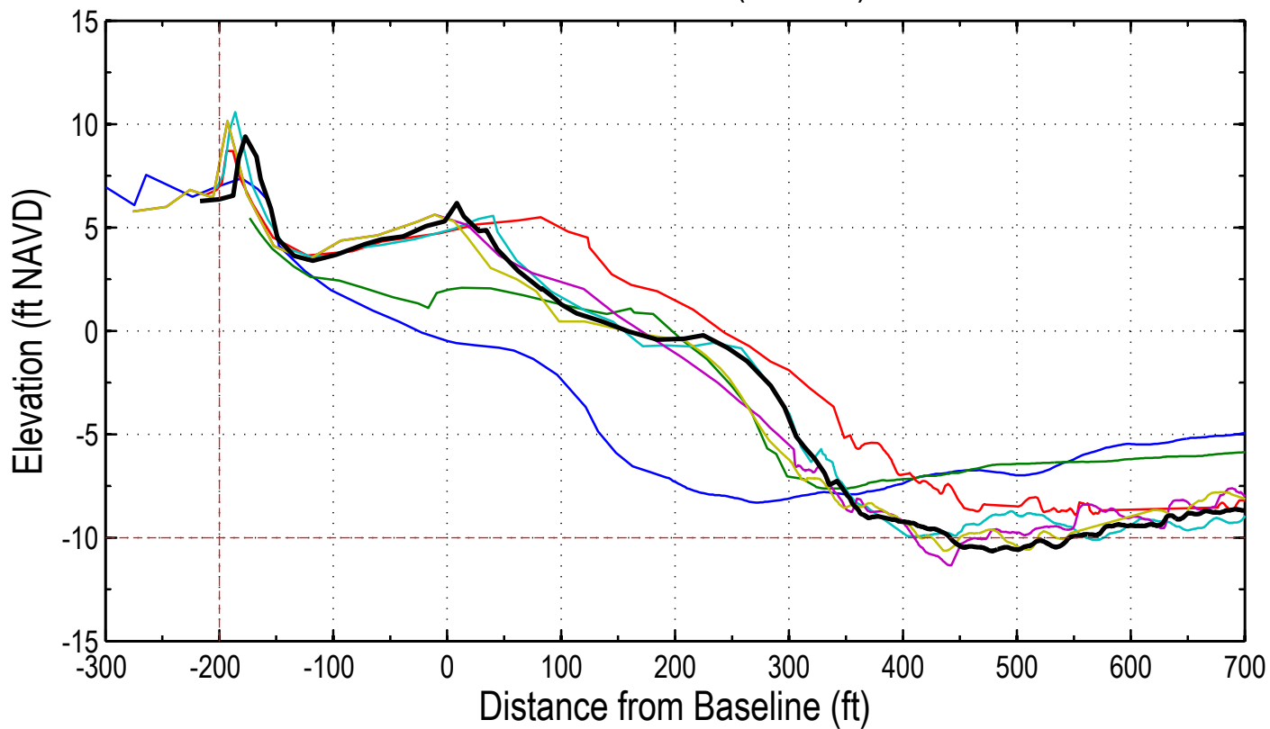
Station: 328+00 (106+00)
